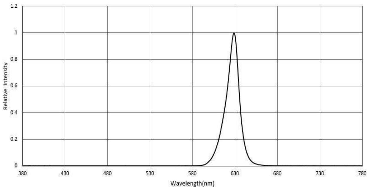
Fig.6 相对光强分布特性曲线
